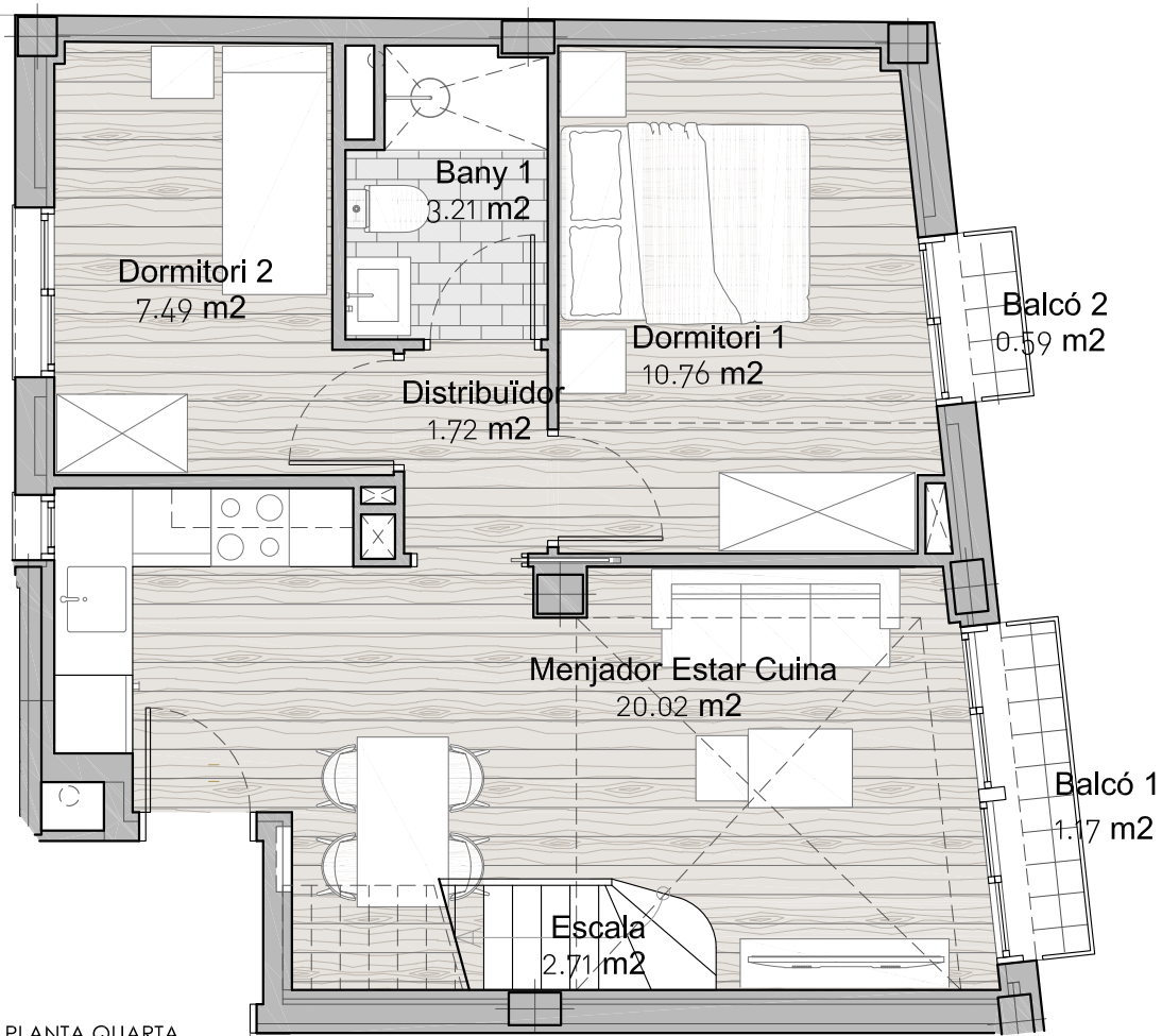
PLANTA QUARTA
