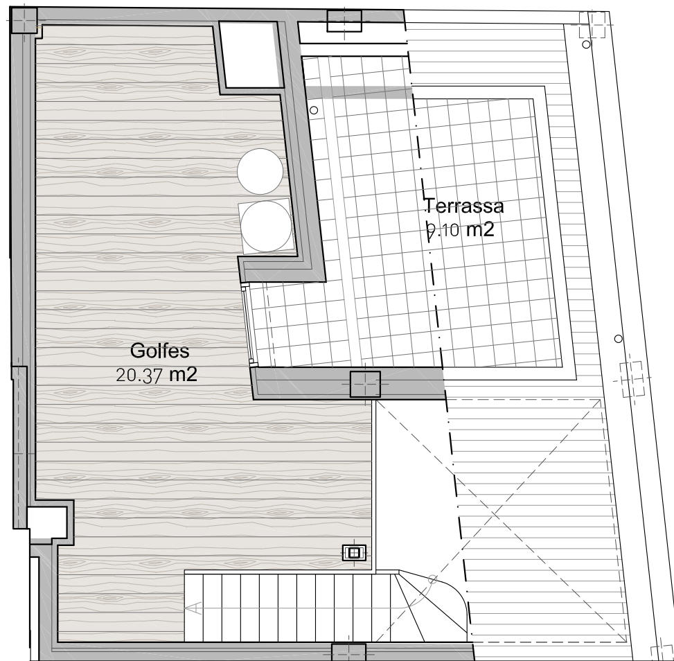
PLANTA SOTACOBERTA
